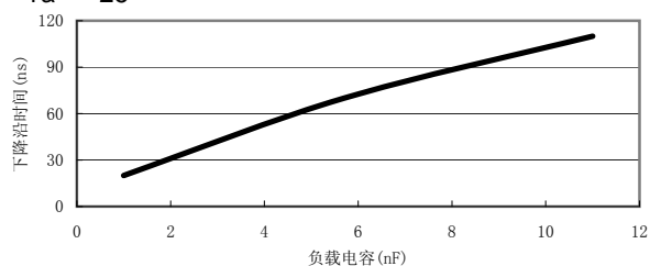
图表2 下降沿时间 vs 负载电容
