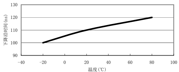
图表6 下降沿时间 vs 温度
