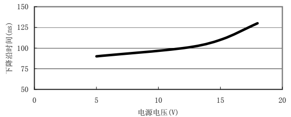
图表4 下降沿时间 vs 电源电压
