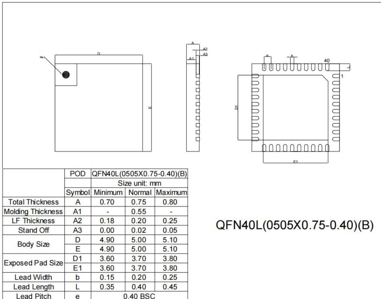
图 5 封装图
