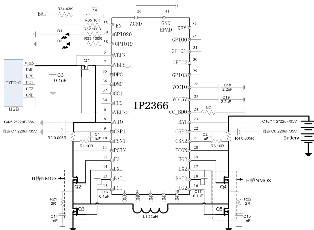
图 4 应用原理图
