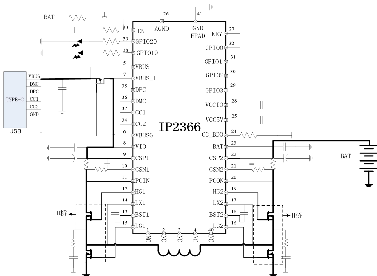
图 1 IP2366 简化应用原理图
