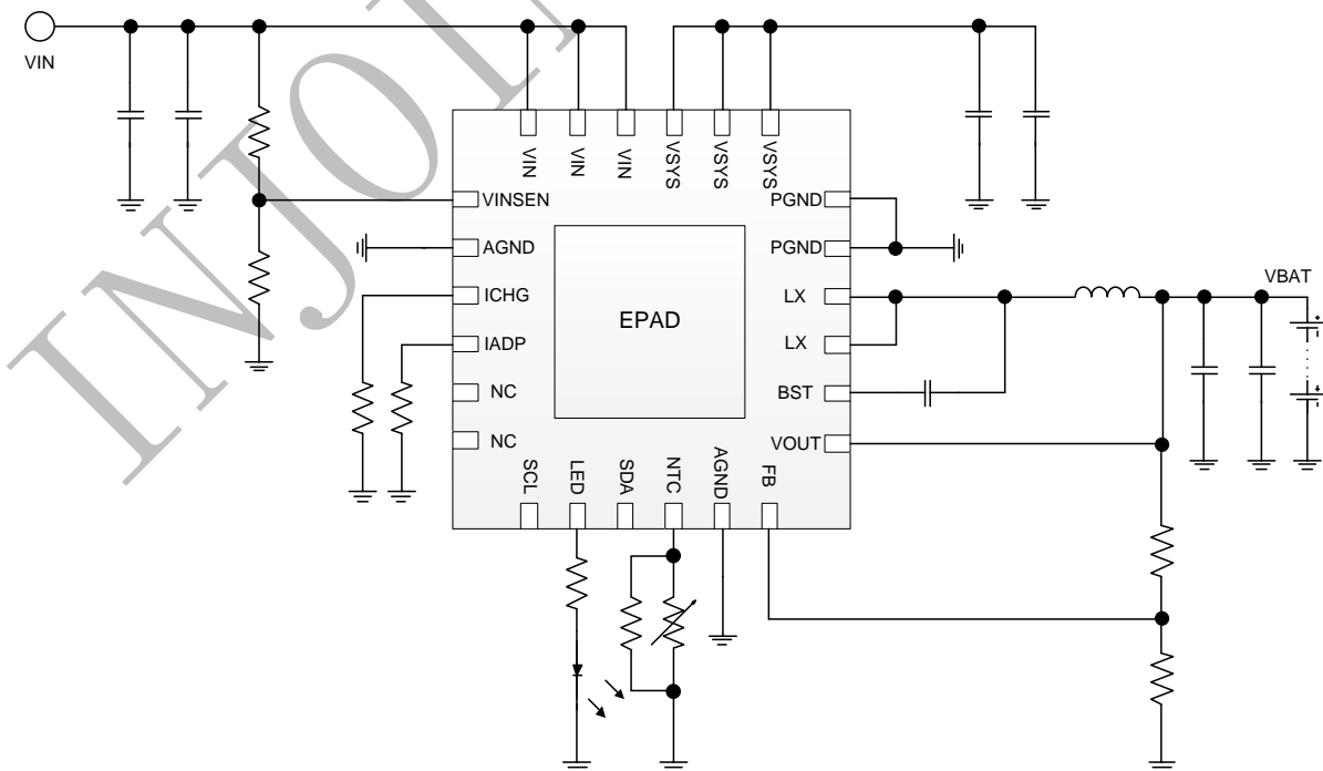
图 1 IP2365 简化应用原理图
