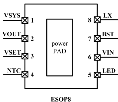
图 2 IP2320 引脚图
