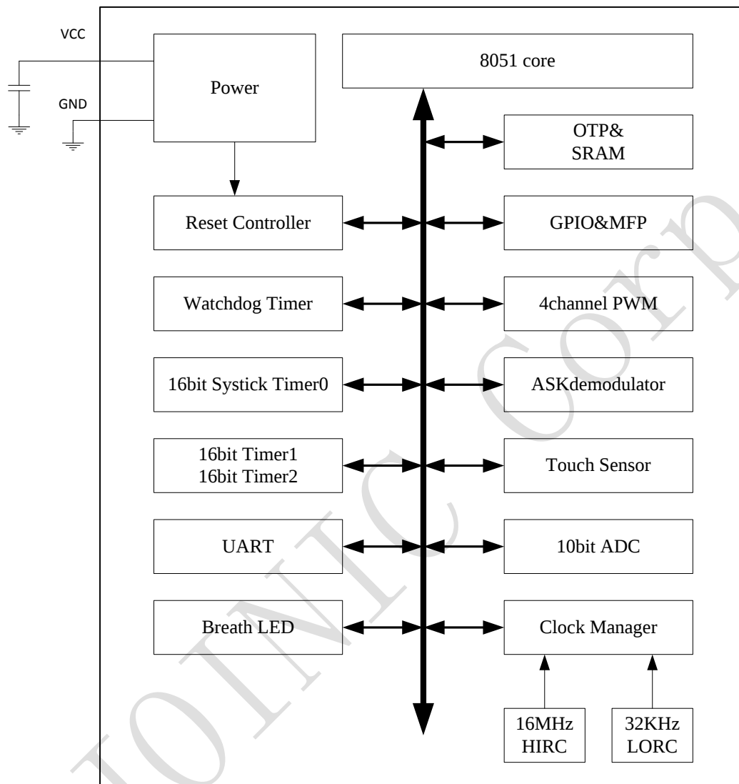
图 3 IP6801 芯片内部框图
