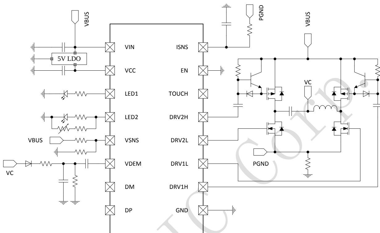
图 1 IP6801 应用原理图
