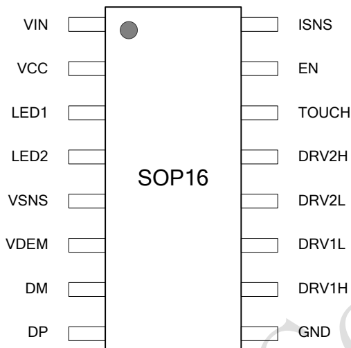
图 2 IP6801 引脚图
