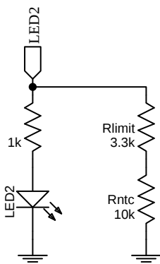
图 5 LED 和 NTC 复用原理图
