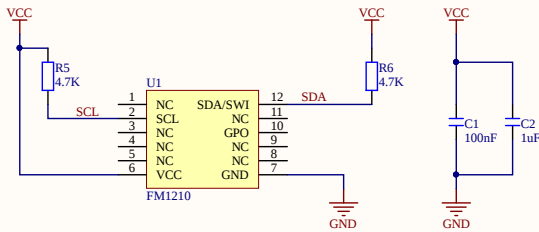
DFN12_I2C 注意:GPO脚不用则悬空
