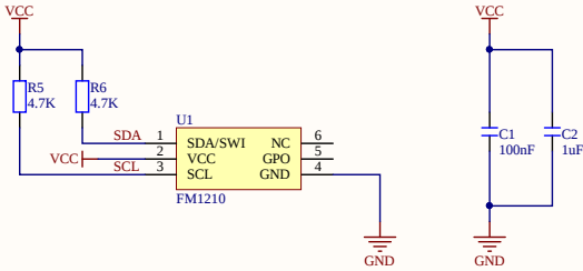
DFN6_I2C 注意:GPO脚不用则悬空
