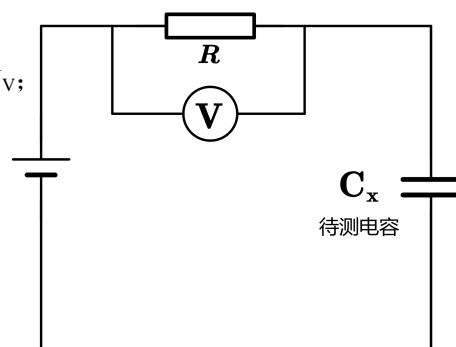
图 4. 漏电流测试电路图
